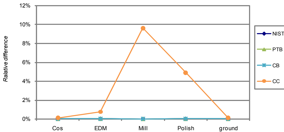
Figure 36: Pdq parameter analysis
