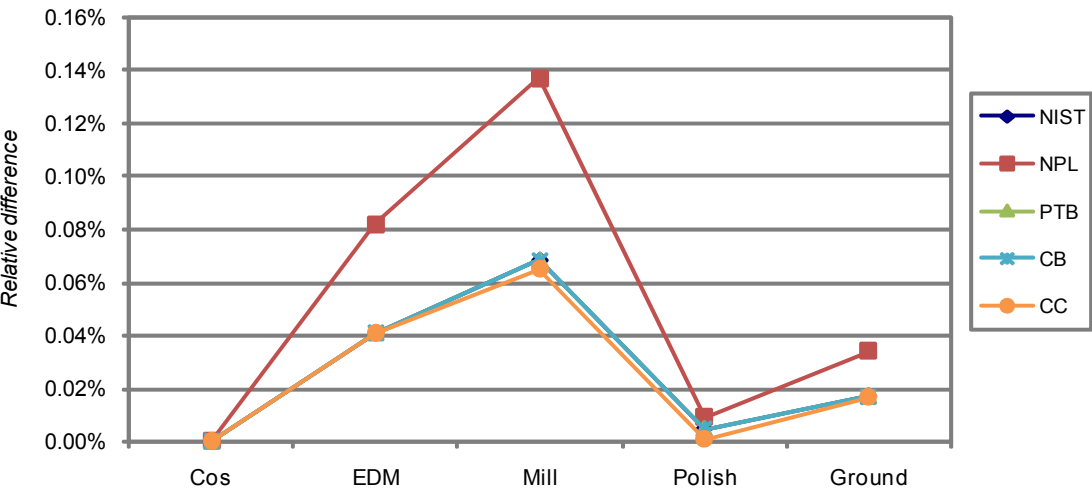
Figure 32: P_t parameter analysis
