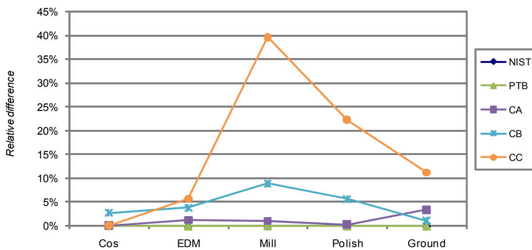
Figure 35: Rdq parameter analysis
