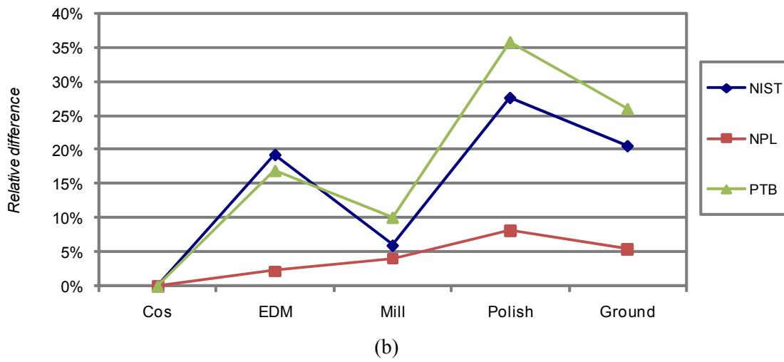
Figure 33: R_{Sm} parameter analysis
