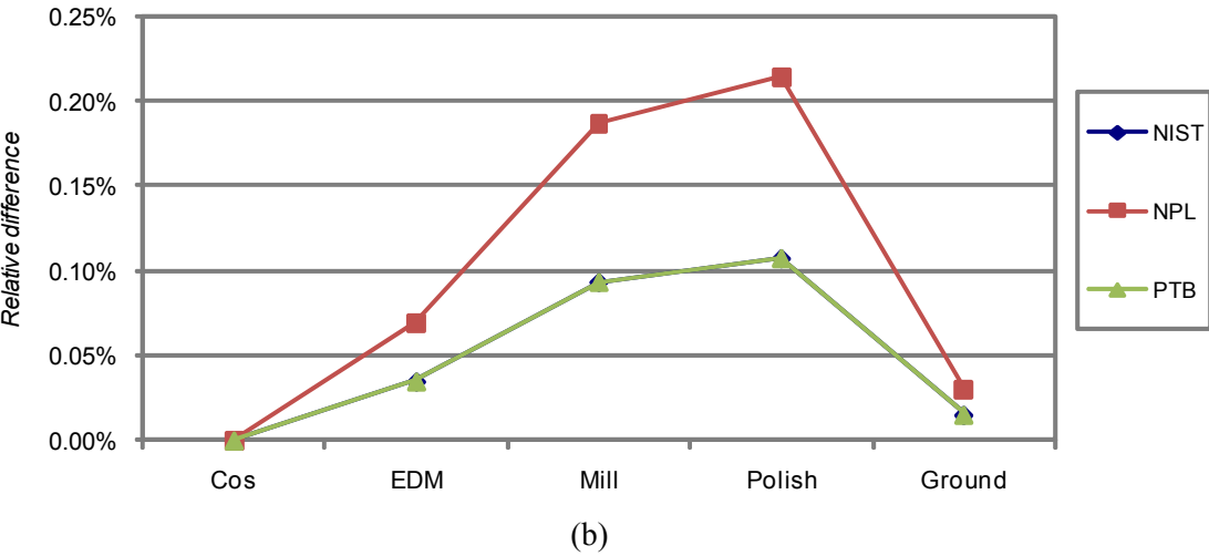
Figure 31: R_t parameter analysis
