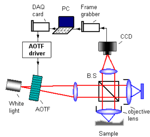
Fig. 1. WSI configuration
